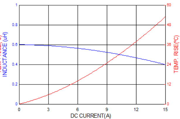
ASPIAIG-F4020-R60
