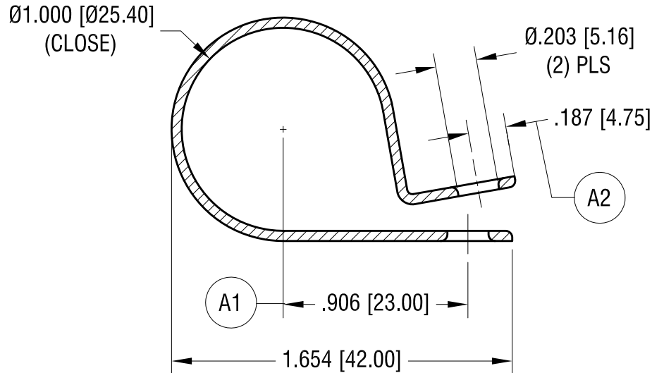
SECTION A-A
